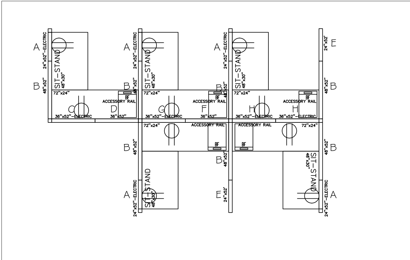
WORKSTATIONS (CUBICLES) GROUPING PLAN PLAN DE REGROUPEMENT DES POSTES DE TRAVAIL (CUBICULES)
