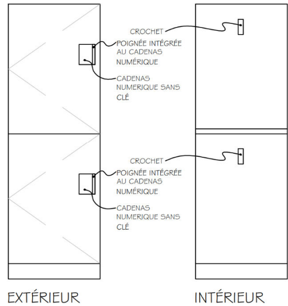
CASIER (DEUX DE HAUT) - 18"
