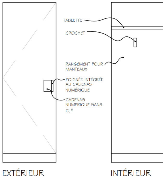
CASIER (UN DE HAUT) - 18"
